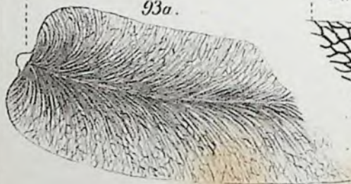
93. Dictyopteris neuropteroides.
