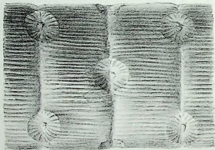
42. C. cruciatus .
