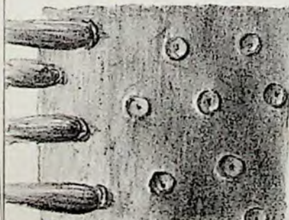
40. Stigmaria ficoides .
