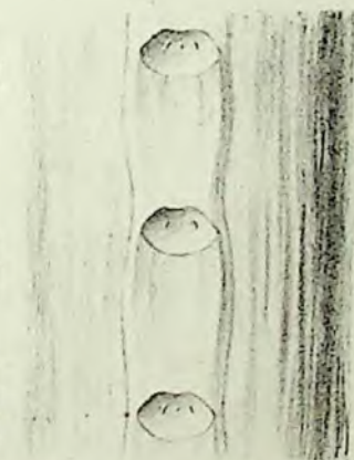
15. S. reniformis .
