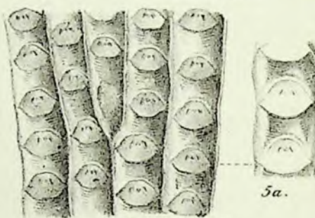
5. S. mamillaris .
