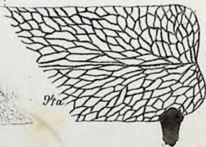
94. Dict. Brongniarti.
