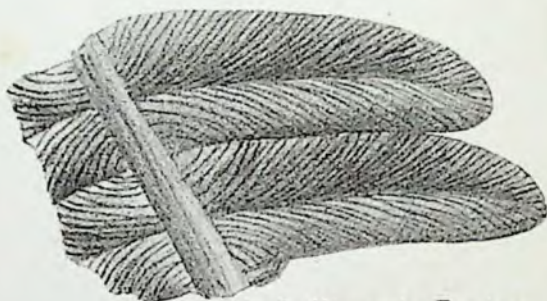
84. Callipteris Regina.
