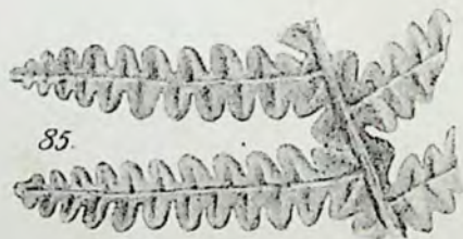
Callipteridium mirabile.
