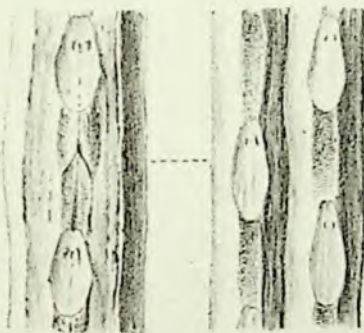
13. S. elongata .
