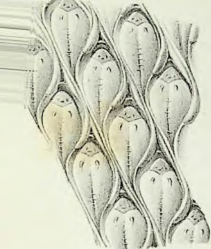
27. L. dichotomum .
