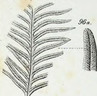
96. Alethopteris Mantelli .
