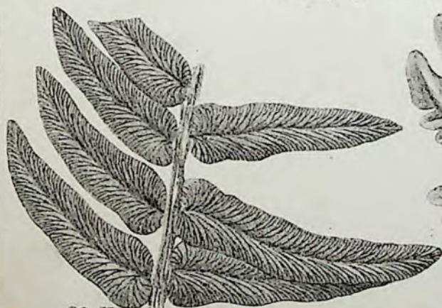
89. N. acutifolia.
