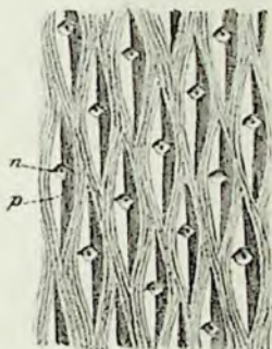
28. L. rimosum .
