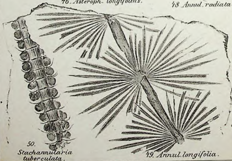
46. Asteroph. longifolius.
