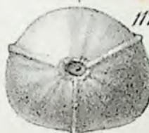
Rhabdocarpus disciformis .
