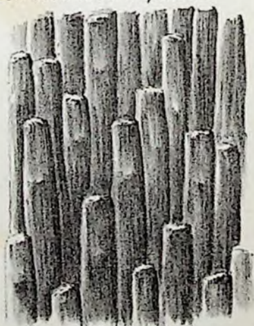
35. Knorria .
