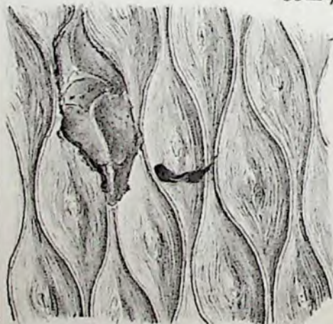
36. Aspidiaria
